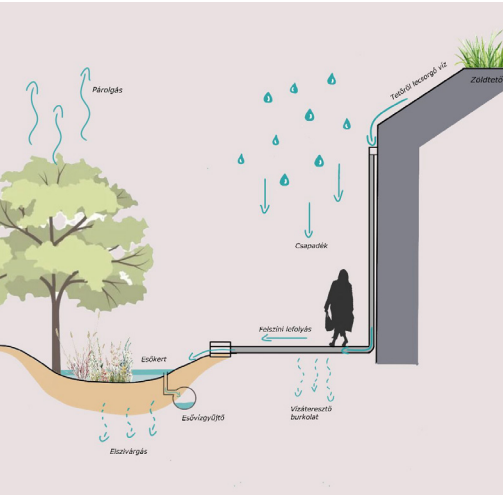
VÍZMEGTARTÁS MÓDJAI (saját szerkesztés, Photoshop)
