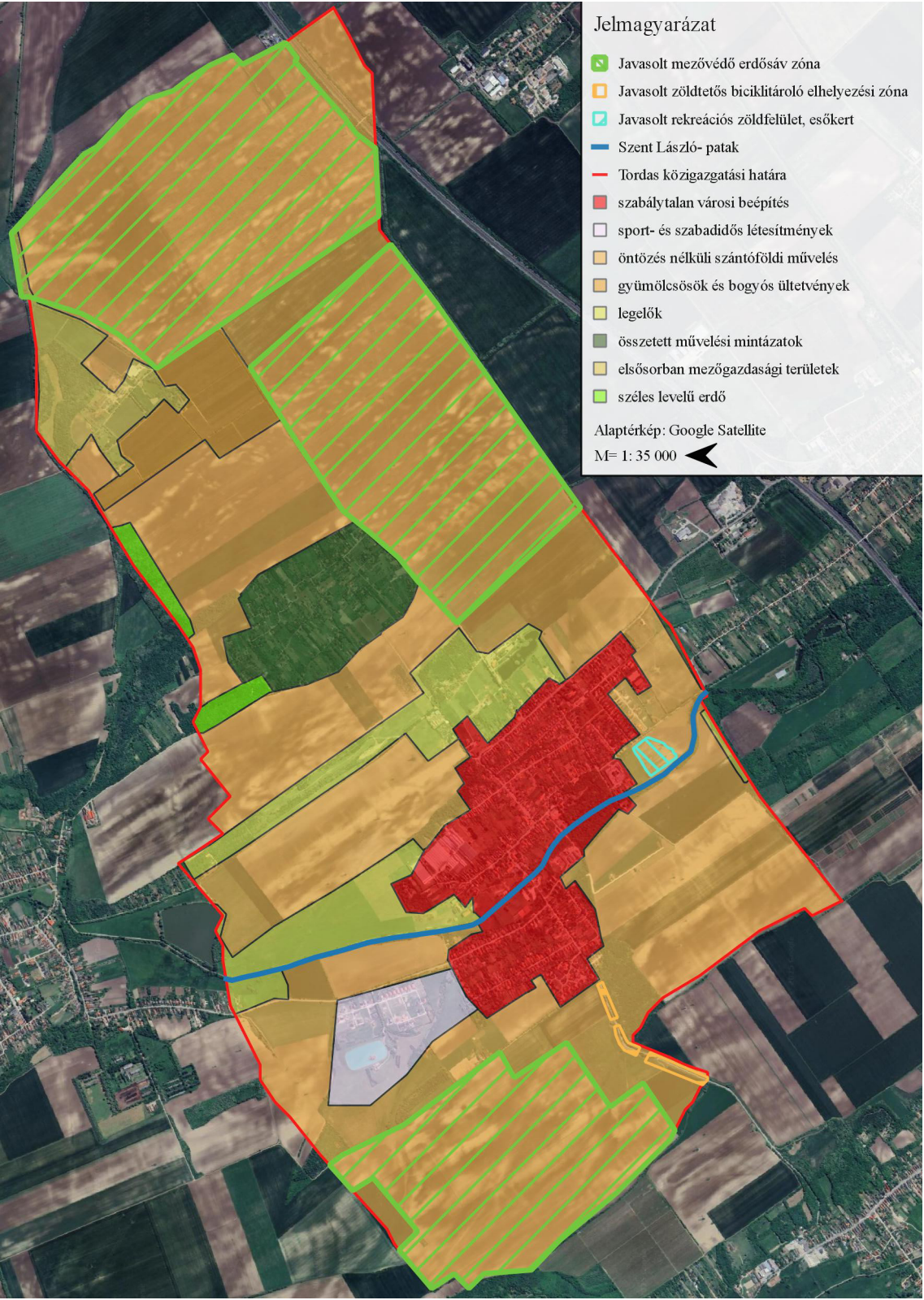
TÁJVIZSGÁLATI TERVLAP (saját szerkesztés, QGIS)
